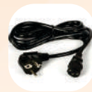
Dây nguồn lõi đồng nguyên chất 2x0.75mmx120cm
